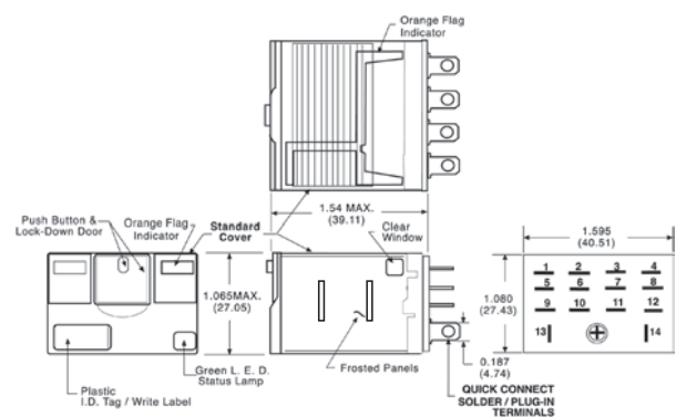
3TX7117 4PDT
