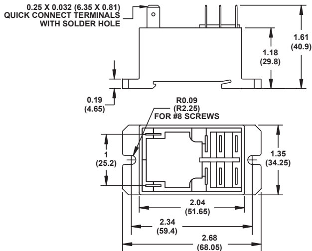
3TX7131 (DPST-NO)
