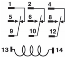
3TX7116 3PDT
