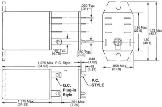
3TX7123
