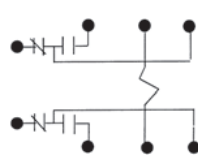
3TX7130 DPDT
