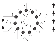
3TX7127 (3PDT)
