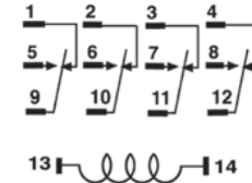
3TX7126/ 3TX7127 4PDT
