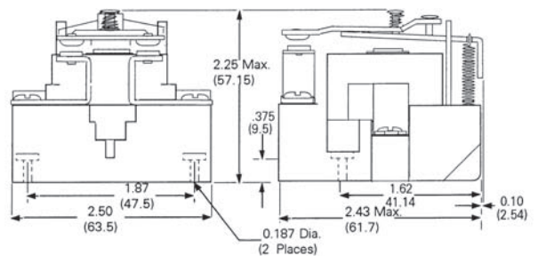
3TX7130 SPST NO
