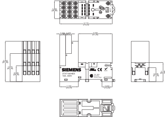
3TX7144-4E5
