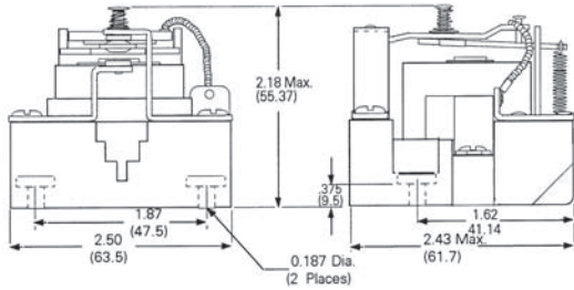
3TX7130 SPDT
