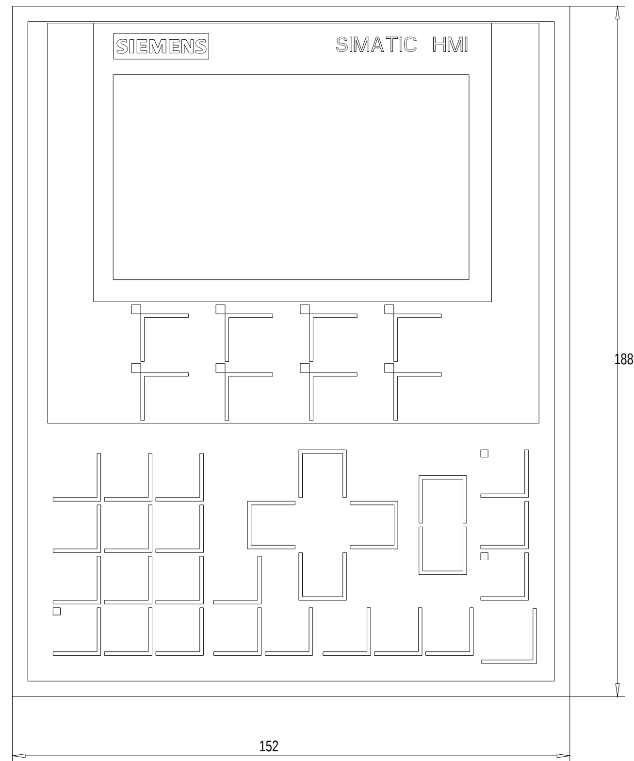
Vorne / Front
