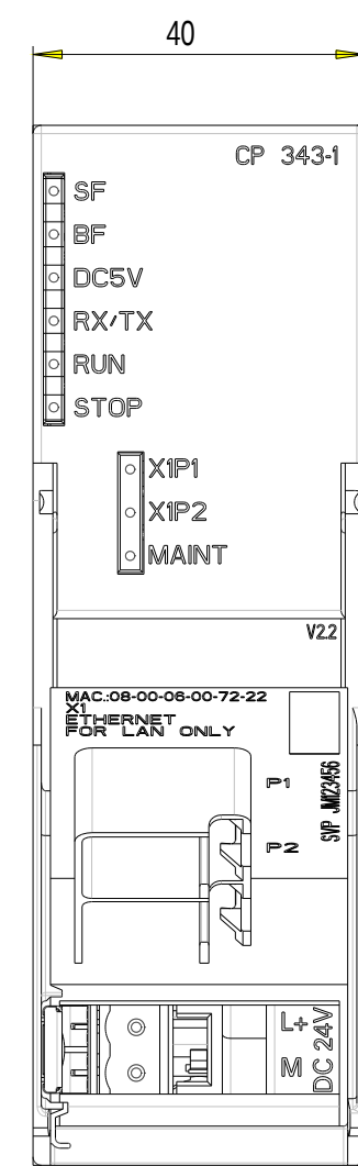
Vorne / Front
